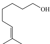
citronellol
